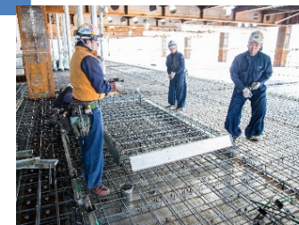
【鋼製型枠を鉄筋上に取付ている作業風景（左が外国人材）】
